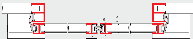
Sezione A – A
